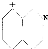
\alpha Säure. Bad. Anilin- u. Sodafabr.
